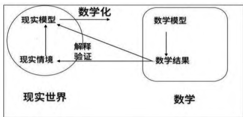
图1 数学建模循环过程
