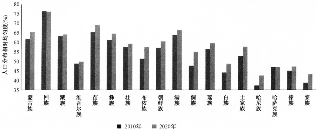
图4 18个百万人口以上少数民族的县级人口分布相对均匀度
