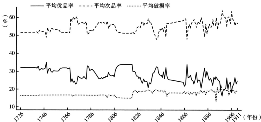
图2 1726-1910年御窑瓷器坯胎优品率、次品率、破损率
